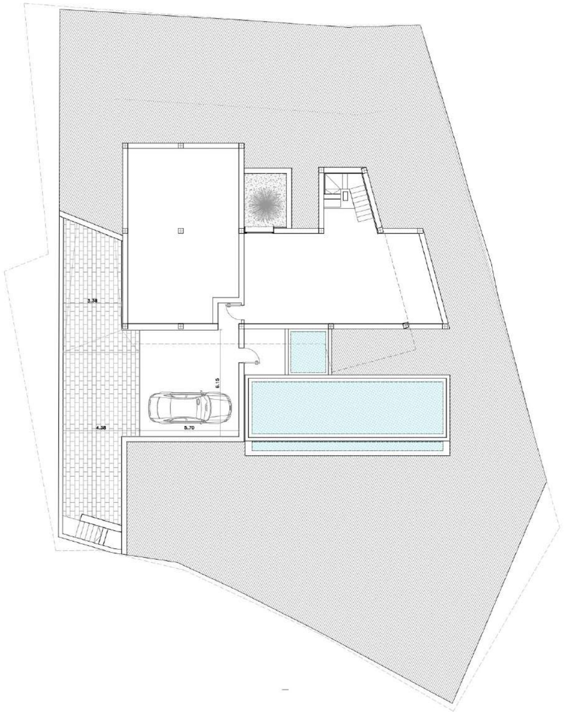
PLANTA SÓTANO
