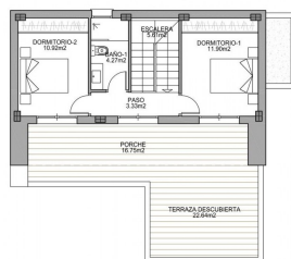
PLANTA PRIMERA
