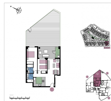
BLOQUE 1 PLANTA B1A VIVIENDA 2
